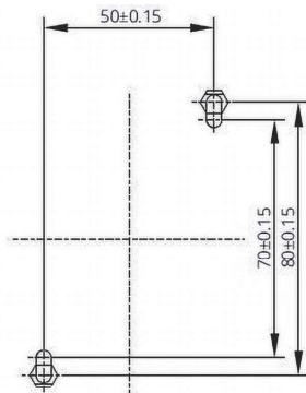
Dima foratura KN43 e KN63
