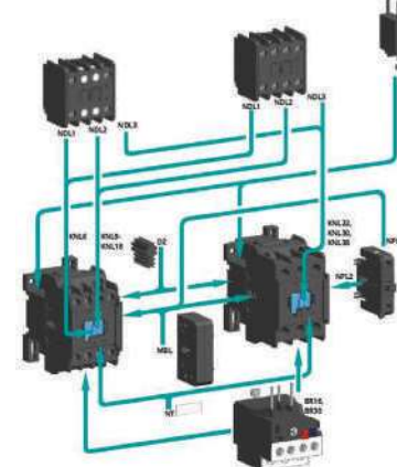
Schema di collegamento
