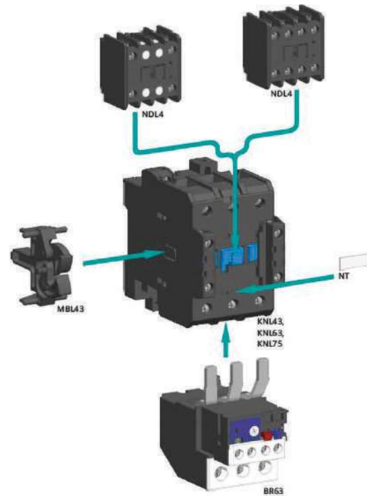
Schema di collegamento
