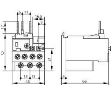
Relè BR16
